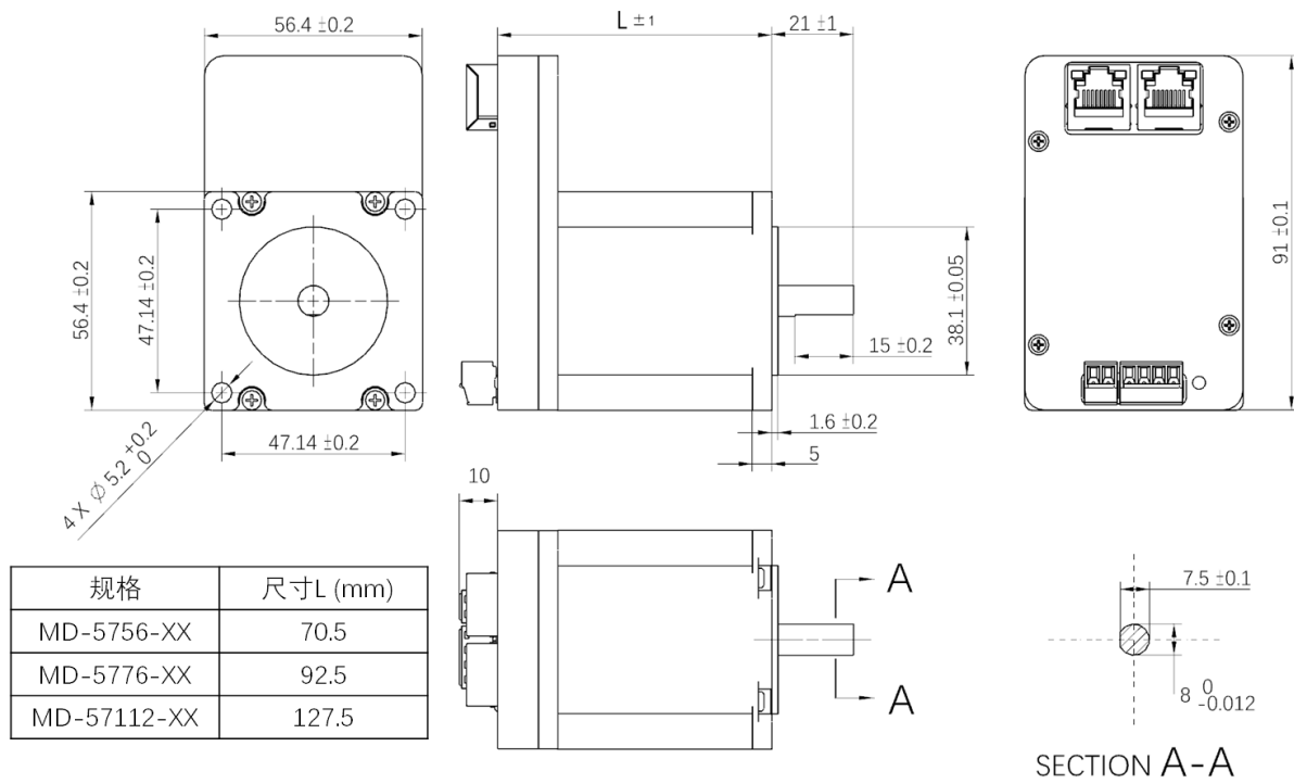
产品尺寸图
