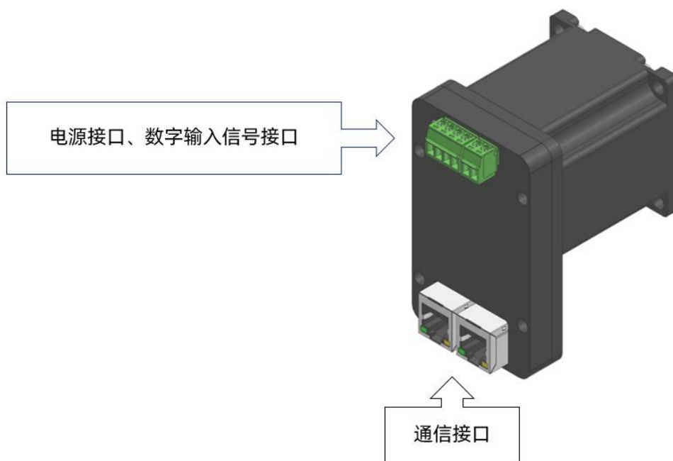
接口示意图
