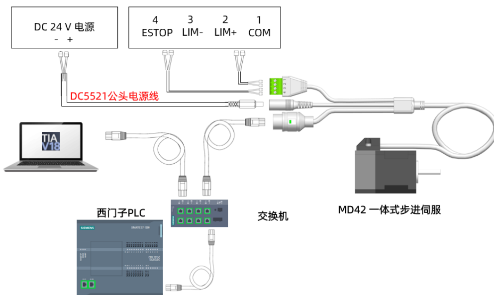
系统连接
